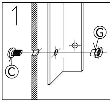
Fijacion de escuadra a lateral Angle plate-lateral locker fixation Fixation de l'équerre au latéral
